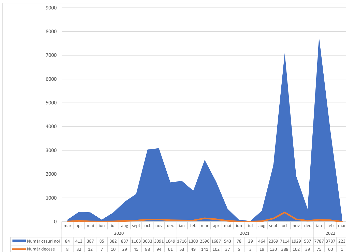
Grafic 1 Cazuri noi și decese COVID-19, 12.03.2020-12.03.2022
